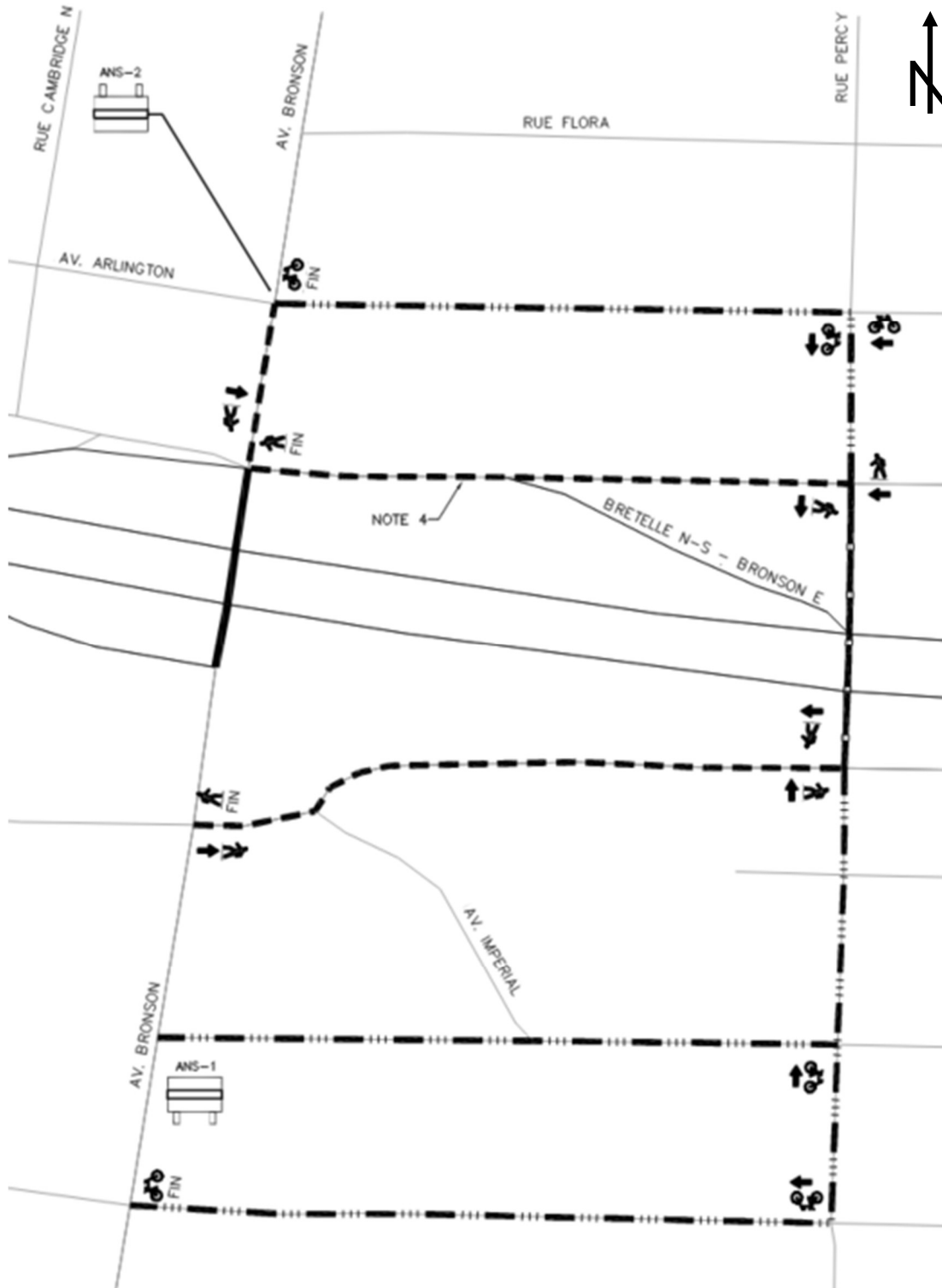
Figure 2 Avenue Bronson – Fermeture entre la rue Catherine et l’avenue Chamberlain – Itinéraire de déviation (piétons et cyclistes)
